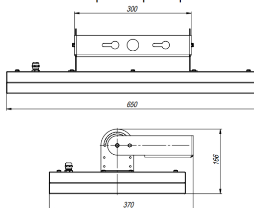
Габаритные размеры
